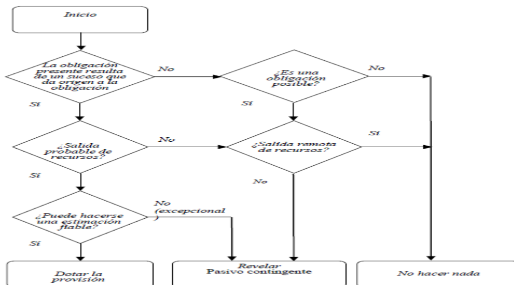
64NICSP 19 ÁRBOL DE DECISIÓN ILUSTRATIVO
